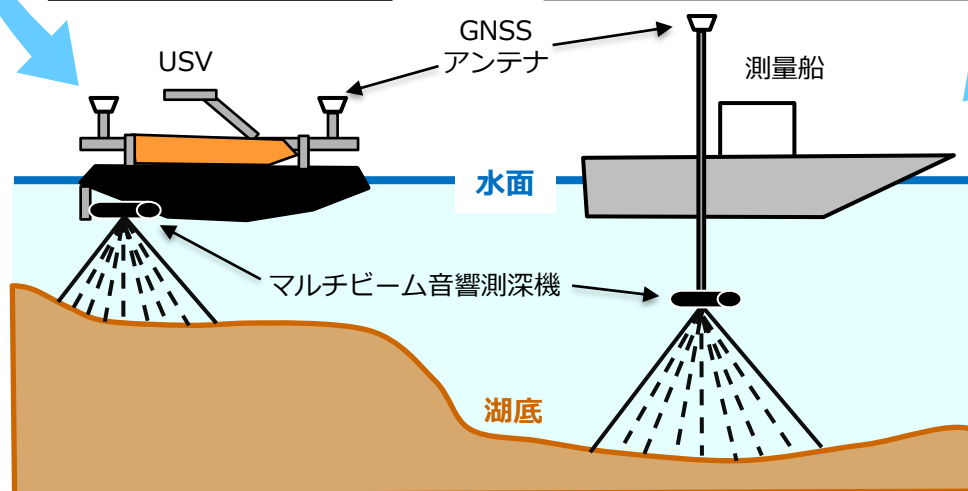
測量計画図のイメージ 小川原湖（青森県）
