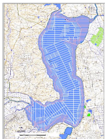
測量計画図のイメージ 小川原湖（青森県）
